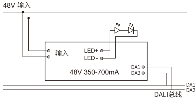
接线图
