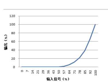
调光曲线
